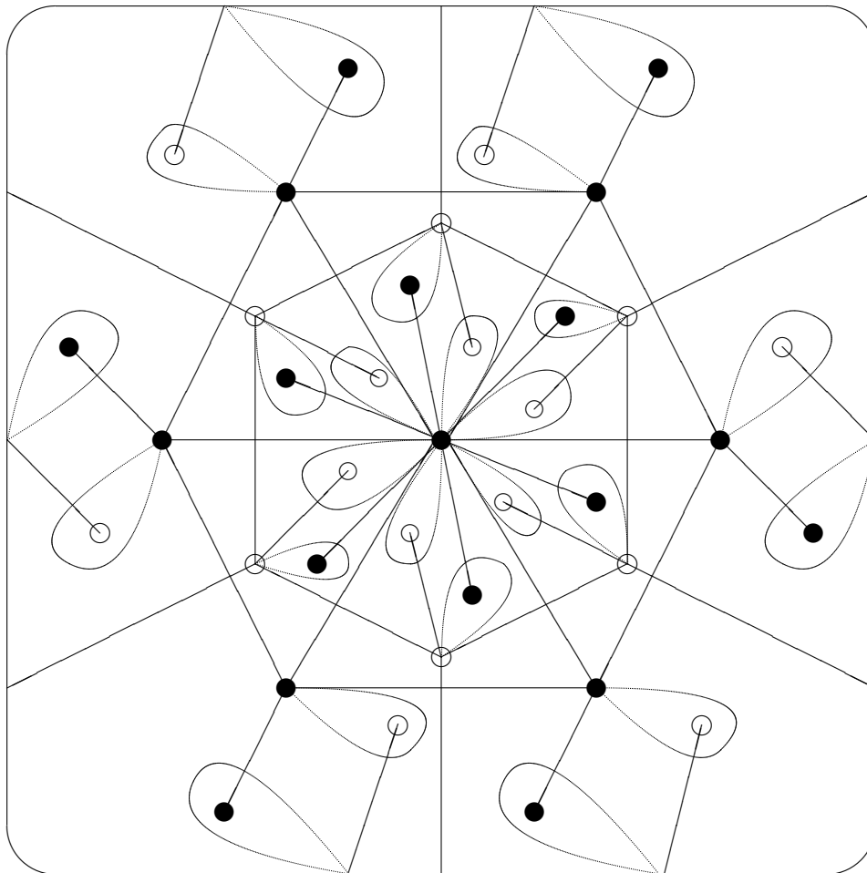
FIGURE 31. [2^+, 12^+] \triangleright [12]^+
